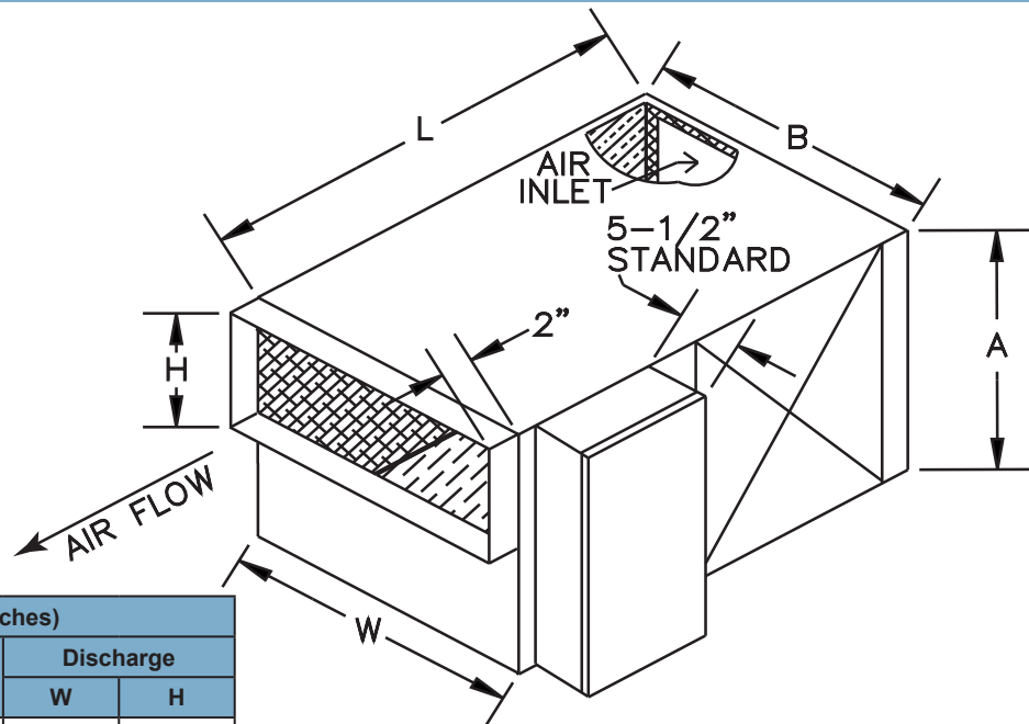
FAN PAC-Electric Heat
